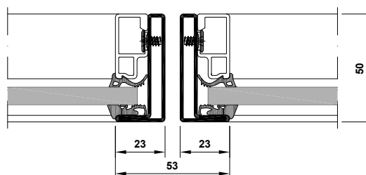
Transition vitrage fixe / vantail de porte
