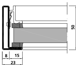
Vitrage fixe
